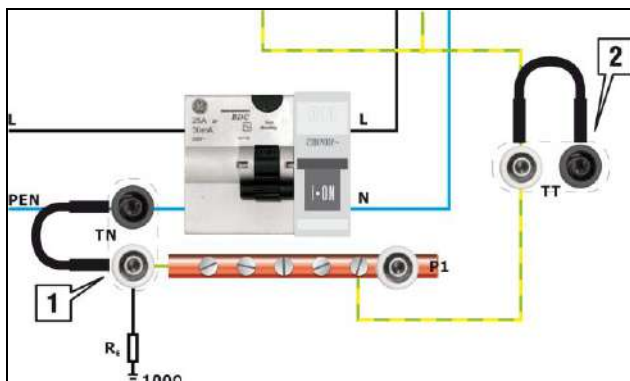
Fig. 3. Puentes de selección del tipo de red. 1 - puente montado que simula las mediciones en la red TN, 2 - puente montado que simula las mediciones en la red TT
