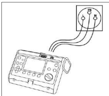
Fig. 6. Conexión del medidor
