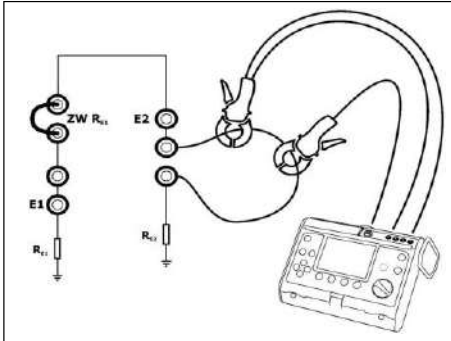
Fig. 11. Conexión del medidor.
