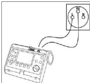
Fig. 19. Conexión del medidor
