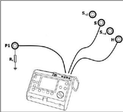
Fig. 7. Conexión del medidor
