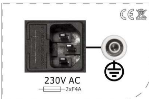
Fig. 20. Colocación de los fusibles
