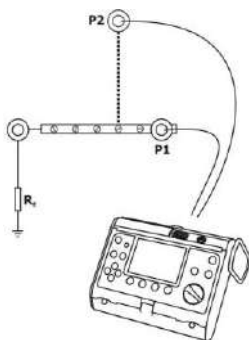
Fig. 16. Conexión del medidor
