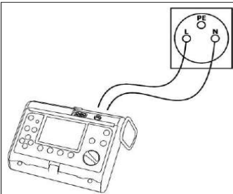
Fig. 18. Conexión del medidor
