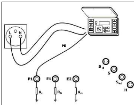
Fig. 12. Conexión del medidor
